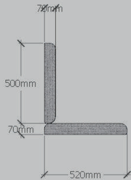
측면도
