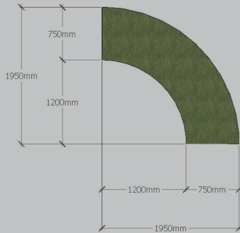
평면도
