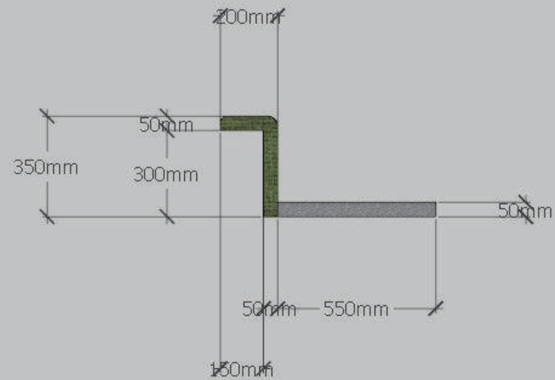
정면도
